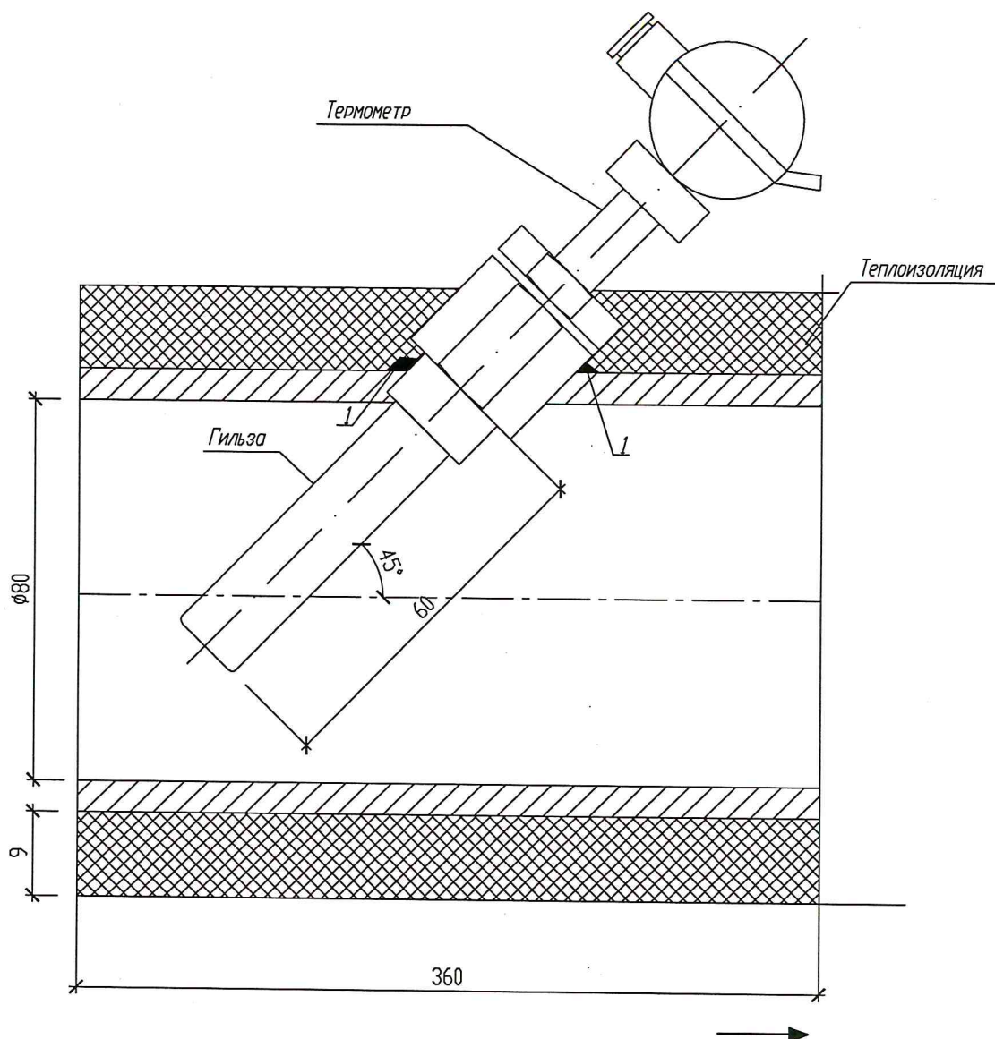
Установка гильзы под КТСРР
